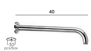
BRAZO REDONDO A PARED Ø2,4x40 cm Material: Latón
