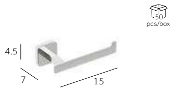
PORTARROLLOS SIN TAPA
