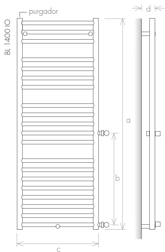
BL1400 IO (in&out) - Ligações laterais
