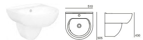
Lavatório . Lavabo . Washbasin 34331XX2C Coluna . Columna . Pedestal . Colonne 34220XX2K
