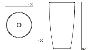
Kobe Lavatório . Lavabo . Washbasin 79910XX2C com saída inferior . %on salida inferior . with bottom outlet . avec sortie inférieure 79911XX2C - com saída lateral . %on salida lateral . with side outlet . avec sortie latérale
