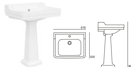
Lavatório médio c/ espaldar .
