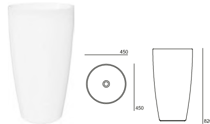
Kobe Lavatório . Lavabo . Washbasin 79910XX2C% com saída inferior . con salida inferior . with bottom outlet . avec sortie inférieure 79911XX2C - com saída lateral . con salida lateral . with side outlet . avec sortie latérale
