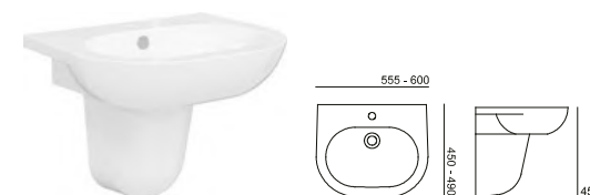
Lavatório . Lavabo . Washbasin 37331XX2C%SC] 37311XX2C%SC]
