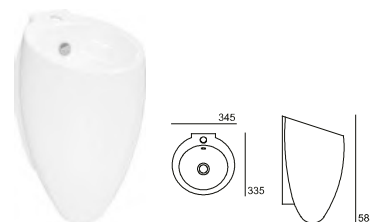
Lavatório . Lavabo . Washbasin 39871XX2K
