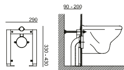
Estrutura de sanita sem tanque . Estructura inodoro sin tanque . Wall-mounted frame toilet without flushing cistern . Bâti-chasse sans réservoir 55036201
