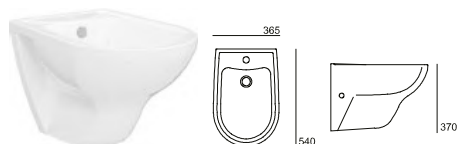
Bidé . Bidet 13401XX2K
